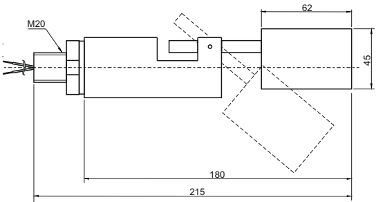
IL-BA-H-P20-P
