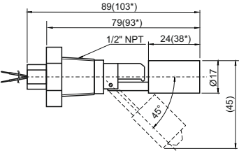
IL-BA-H-P1/2NPT-P(IL-BA-H-P1/2NPT-F)
