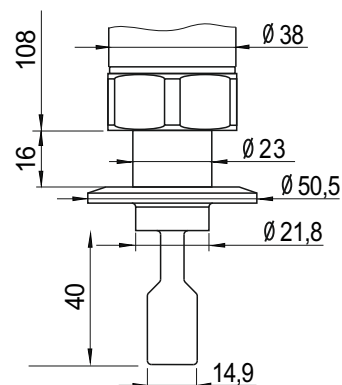
Версия с соединением Clamp DN40 зонд 100мм
