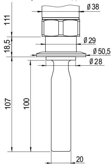
Версия с соединением Clamp DN40 зонд 100мм
