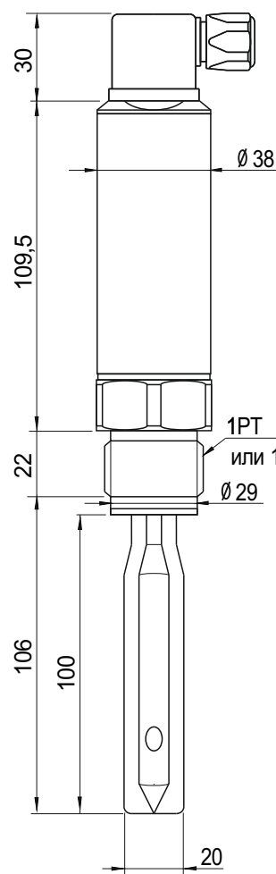
Версия с резьбой 1" и разъемом DIN 43650
