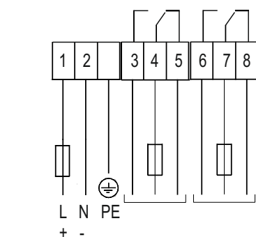
Источник питания Выходной сигнал
