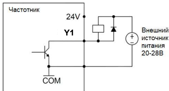
Рис.3-13 Способ подключения внешнего источника питания
