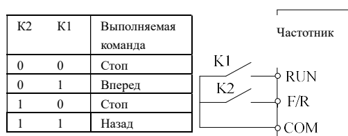
Рис. 6-14 Двухпроводной режим управления 2
