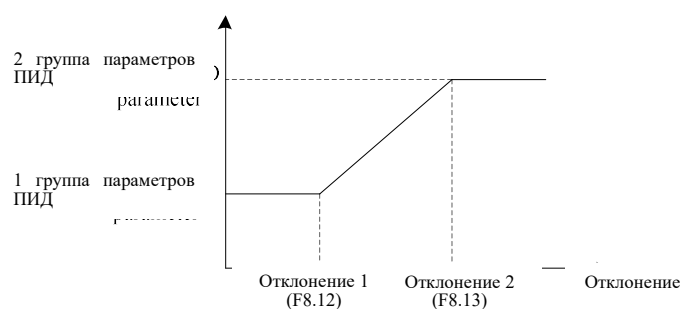
Рис. 6-23 Переключение параметров ПИД
