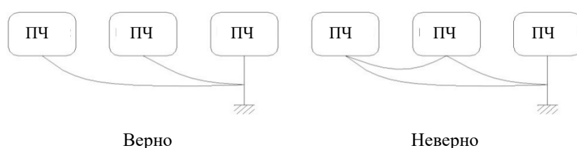
Рис. 3-5 Заземление
