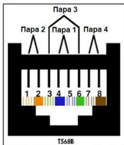
Рис. 3-15 Стандартный T568B
